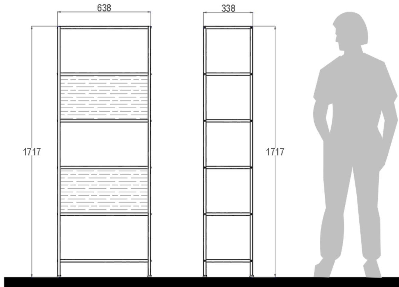
ALZADO FRONTAL
