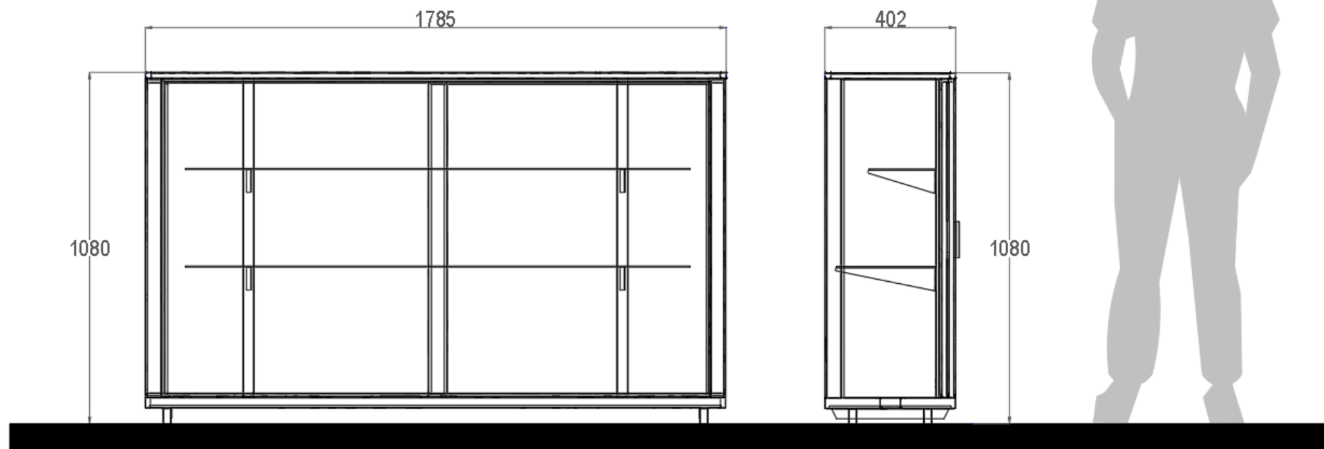
ALZADO FRONTAL
