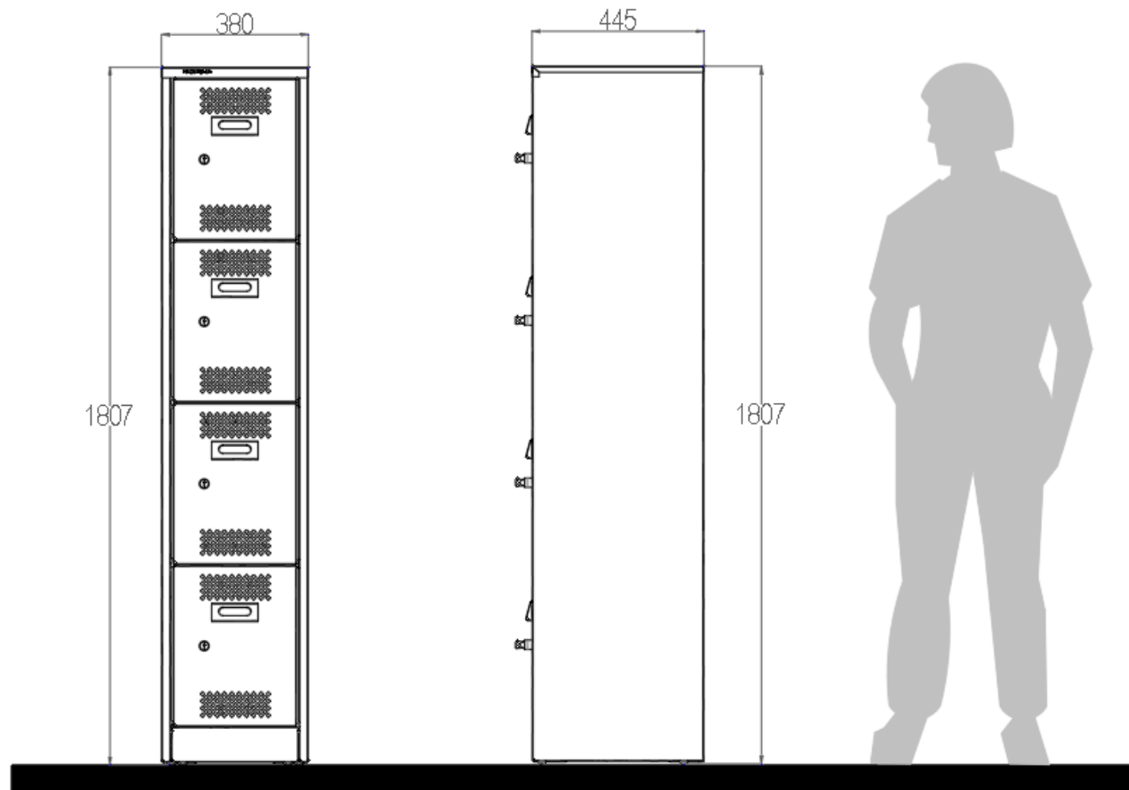
ALZADO FRONTAL
