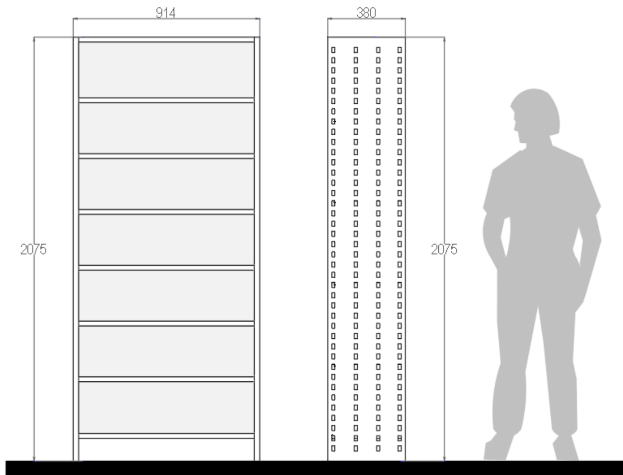
ALZADO FRONTAL
