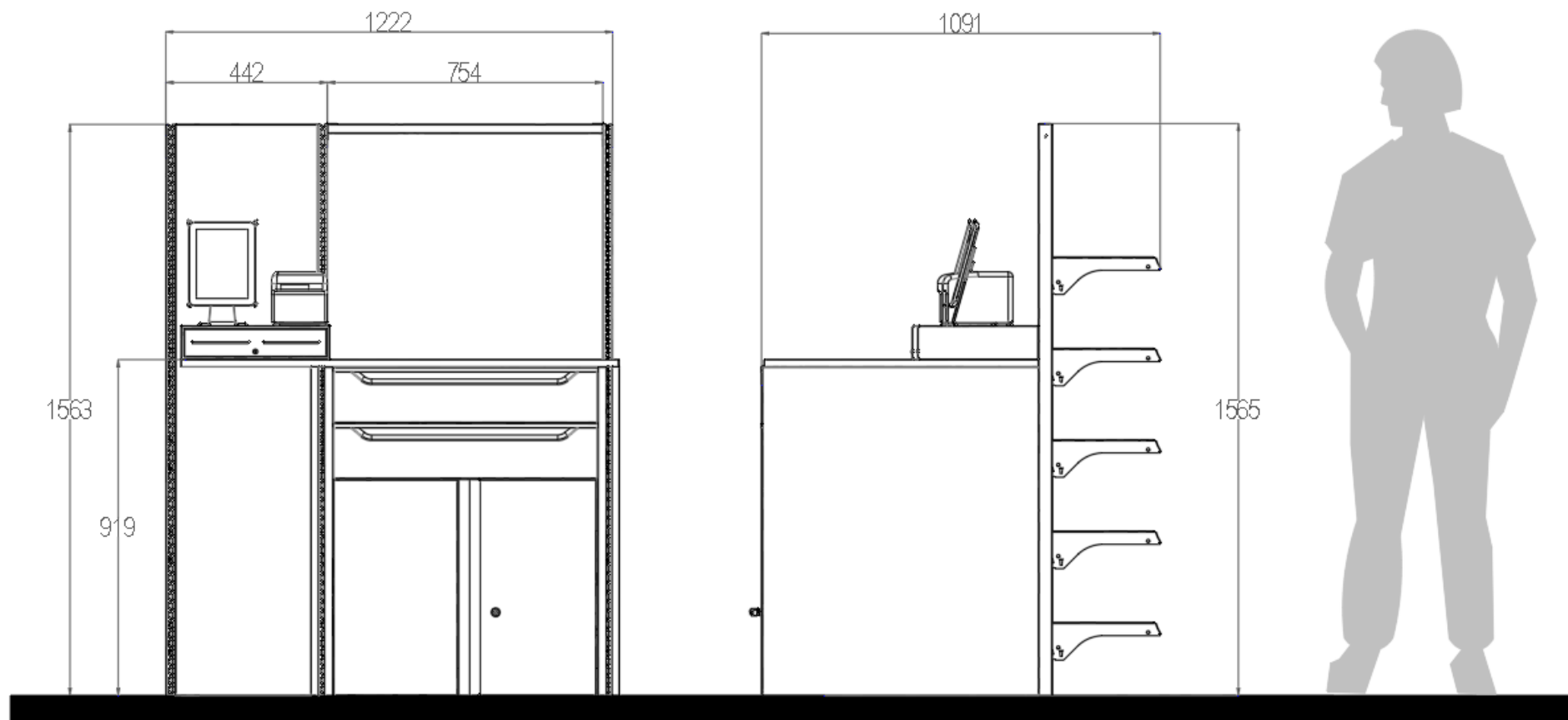
ALZADO FRONTAL
