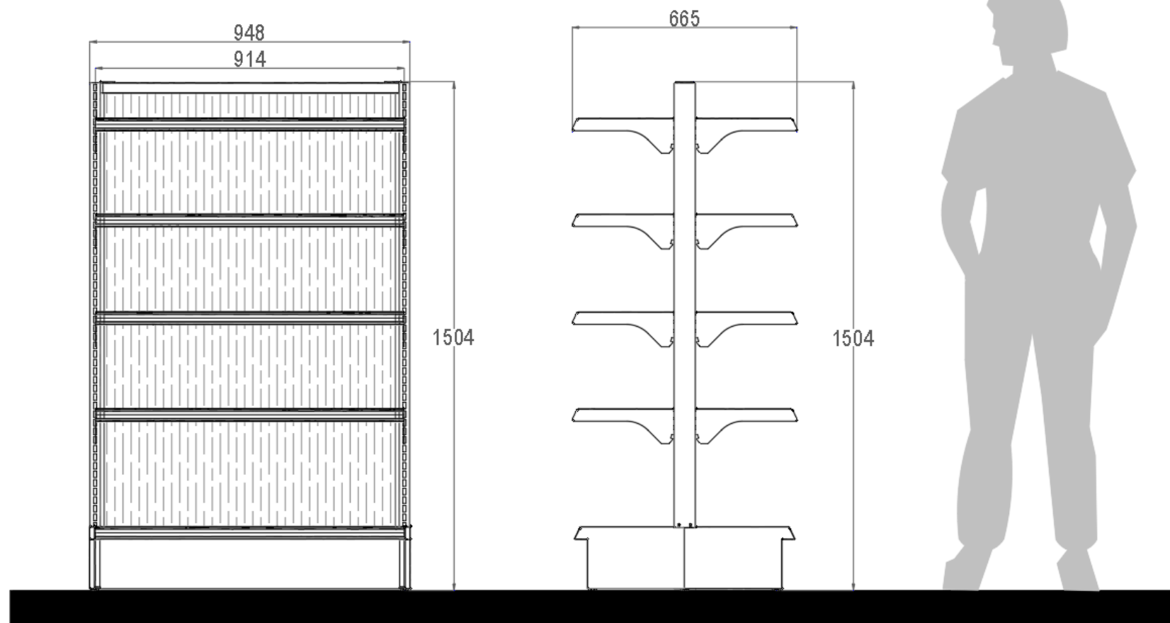
ALZADO FRONTAL
